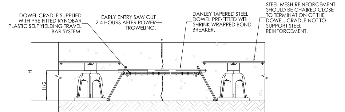
SAWN DOWEL JOINT (S.D.J.) SCALE: 1:8
